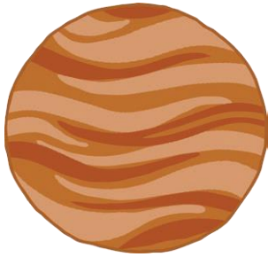
Jupiter
